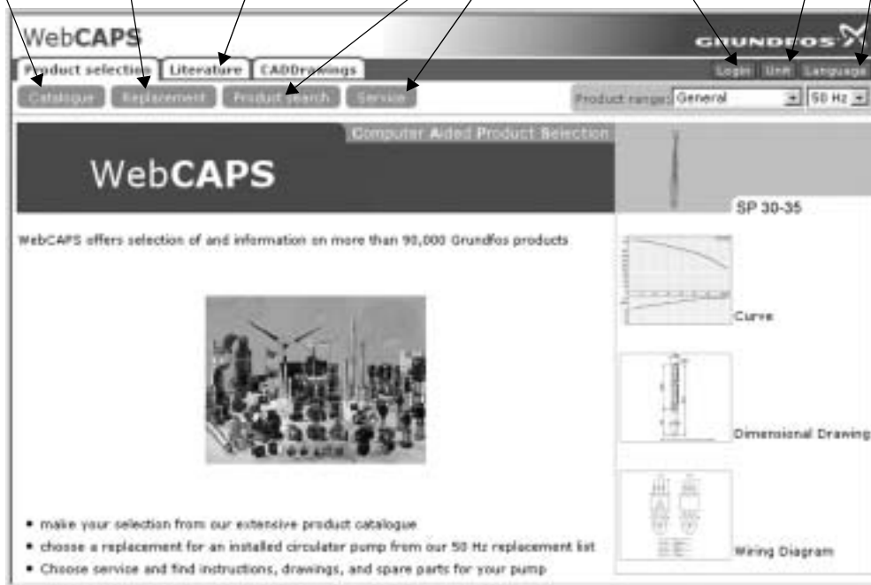
Рис. 30 WebCAPS
